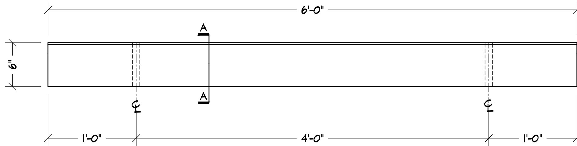
CURB ELEVATION SCALE: 1 1/2" = 1'-0"
