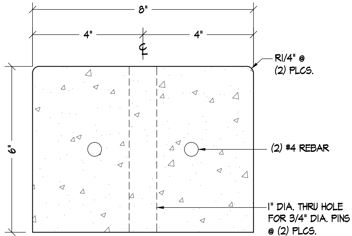
SECTION "A-A" SCALE: HALF
